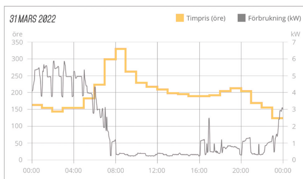
Exempel på hur Ngenic Tune minskar förbrukningen automatiskt när elpriset är högt.
