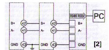
(2) Anslutning till RS485 datanät RS485 koppling med CAT5 kabel: 41 - A - Vit/Grön 42 - B - Grön 43 - GND - Blå
