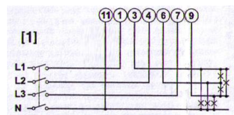
(1) Anslutning till 3 fas elnät
