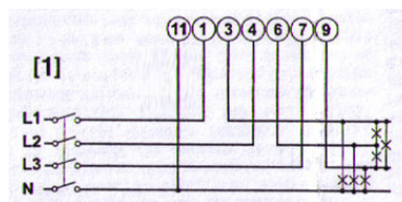
(1) Anslutning till 3 fas elnät
